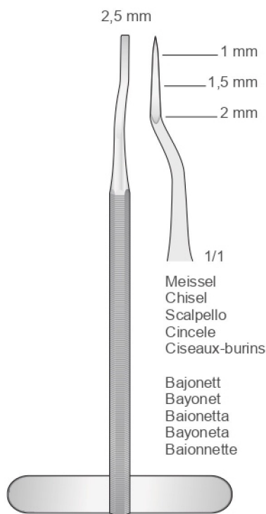
DI-DL-89 130 mm
