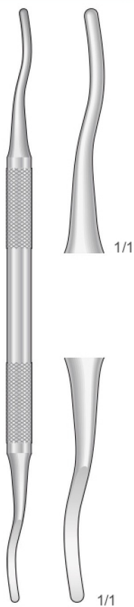
HOPKINS DI-718-191 185 mm
