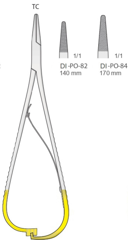
MATHIEU DI-PO-82/ DI-PO-84
